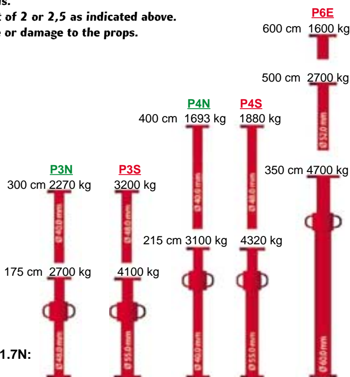
EKSEMPEL PÅ BRUK AV FERMAR DEKKESTØTTER, SKRÅSTØTTER OG PFEIFER FORSKALINGSBJELKER PÅ BYGG
